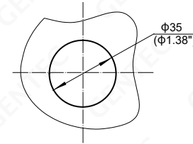
面板安装尺寸图 (最厚7 mm)
